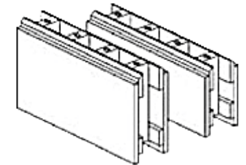
BaKo Grundmodul 4-teilig Länge 640 mm Höhe 320 mm, 240 mm
